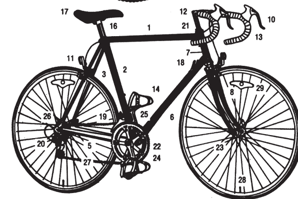
Рис. 4 Дорожный велосипед
